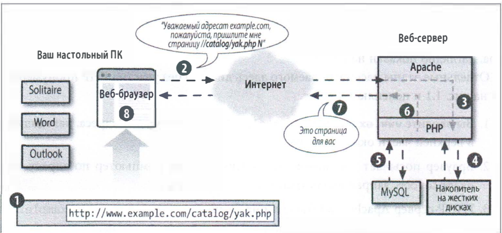
Рис. 1.2. Связь клиента с сервером при участии PHP
