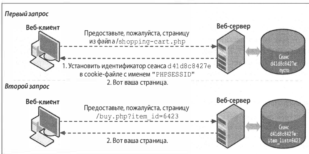
Рис. 10.2. Взаимодействие клиента и сервера вначале сеанса
