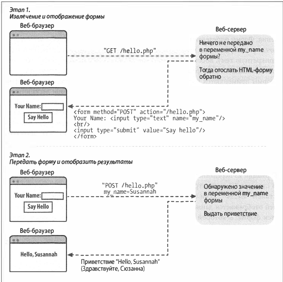
Рис. 7.1. Отображение и обработка простой формы
