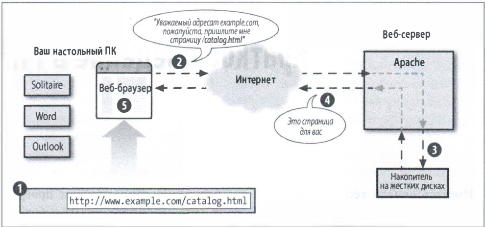
Рис. 1.1. Связь клиента с сервером без участия PHP
